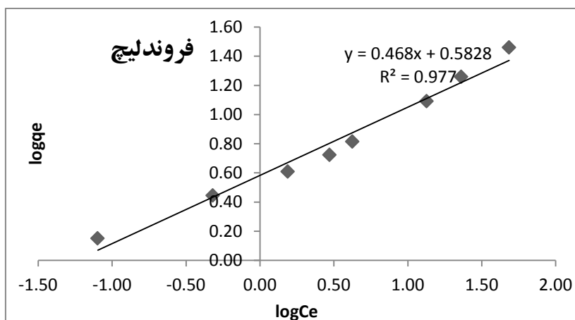
شکل ۳: ایزوترم فروندلیچ جذب رنگ آبی ۷۱ بروی جاذب معدنی پامیس، در دمای ۲۵ درجه سانتی گراد
