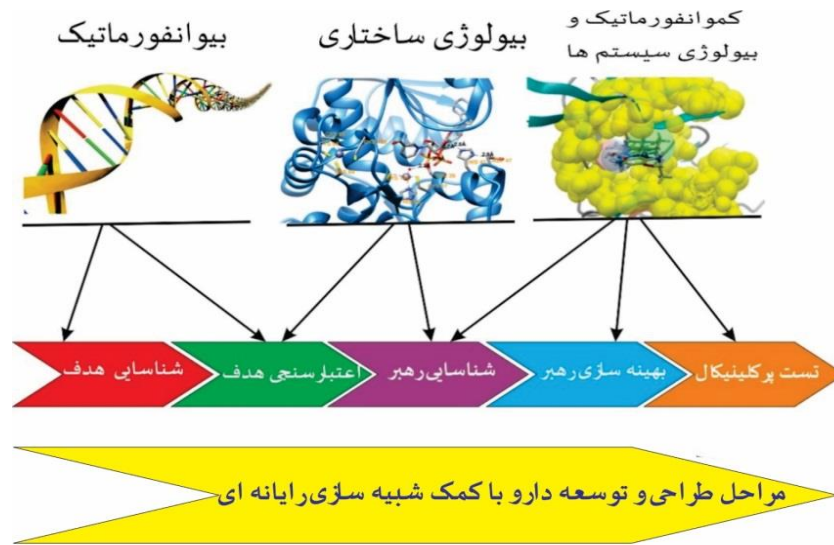
شکل ۲: نمای شماتیکی از مراحل طراحی دارو بوسیله تکنیک‌های مختلف in silico
