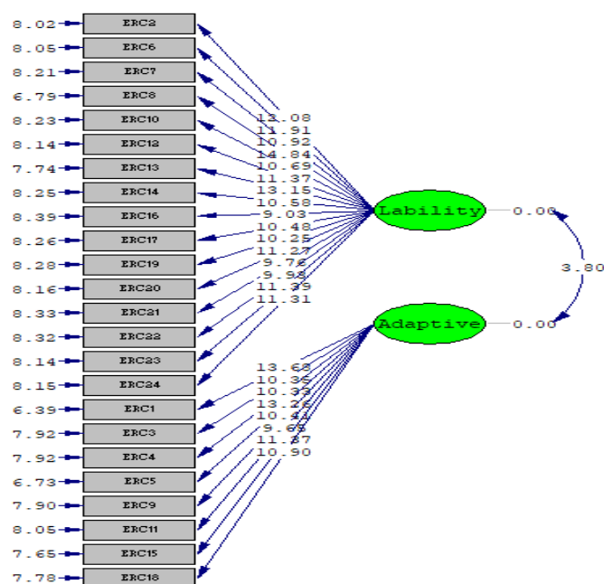
شکل 3: مقدار t-value
