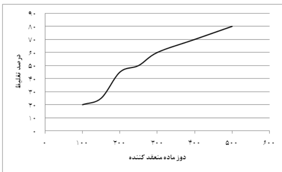
نمودار ۳: درصد تغلیظ لجن در غلظت‌های متفاوت کلریدفریک
